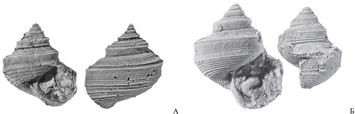
Рис. 5.39. Казанский ярус. Гастроподы (слепки раковин): А – Baylea burtasorum , Кировская обл., Татарстан; Б – Biarneaspira angulata ; Татарстан (по: Мазаев, 2016, 2017).
