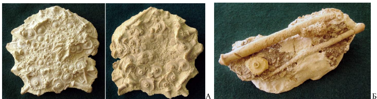
Рис. 4.78. Мелеховский горизонт. Иглокожие: морской ёж Archaeocidaris rossicus . А – давленый панцирь, Соколы горы; Б – иглы и пластинка, Губинские высоты. ИЭВБ, фото Д.В. Варенова.
