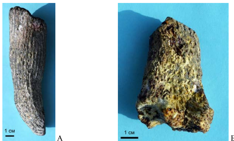
Рис. 8.48. Сенгилейская свита. Кремниевые губки: А – Sororistirps tubiforme , Б – Rhizopoterion cervicorne , фосфатизированные скелеты. Разрез Подвалье. ИЭВБ, фото В.П. Морова.
