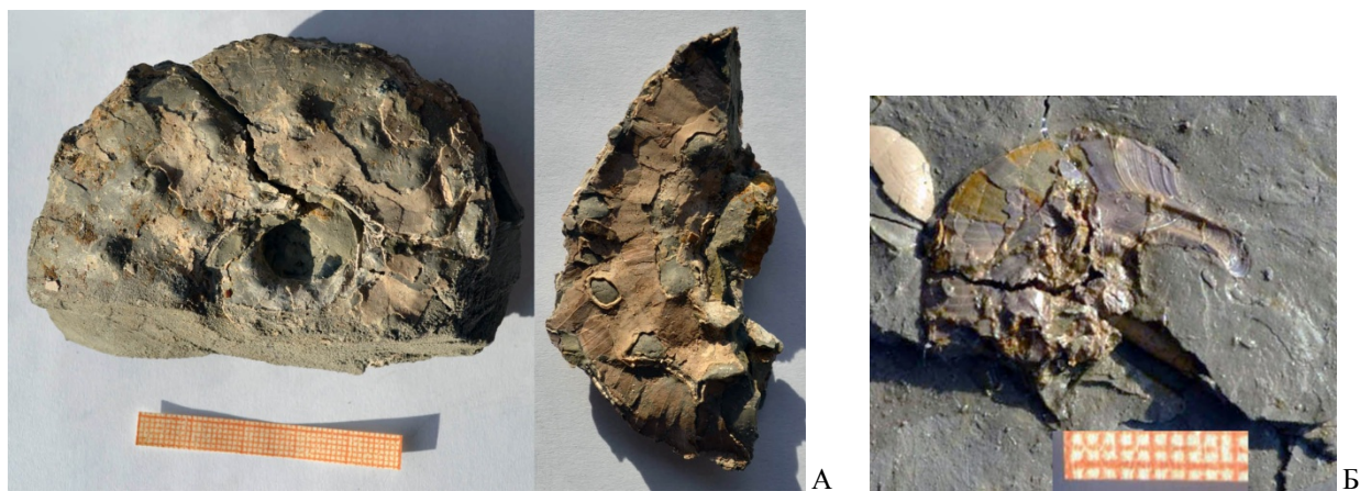
Рис. 7.36. Верхний кимеридж. Аммониты: А – Aspidoceras cf. catalaunicum , ядра с остатками раковин; Б – Sutneria perplexa , устье раковины. Гор. Сызрань. ИЭВБ (А), ГИН (Б); фото В.П. Морова.
