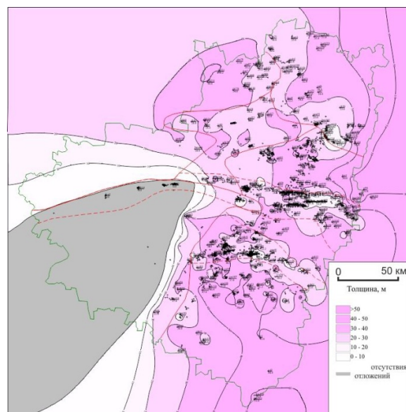
Рис. 3.32. Доманиковый горизонт. Распространение и мощность (по: Потёмкин, 2015).
