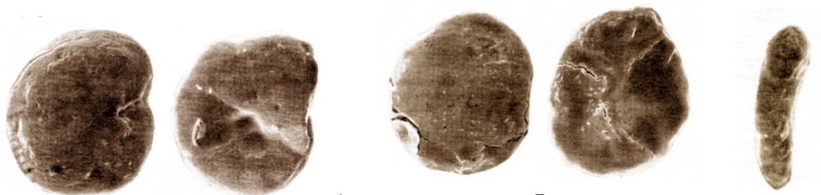
Рис. 8.18. Уренская толща. Фораминиферы: А – Gyroidina sokolovae , Б – Serovaina barremica , В – Gaudryinopsis filiformis , раковинки (сильно увел.), разрез Форфос (Сызранский р-н) (по: Барабошкин, 2001).
