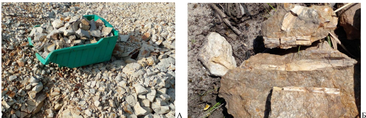
Рис. 9.20. Камышинская свита: А – ошеснённый слой опок с гнездообразными включениями диатомитов/трепелов, ур. Осиновка (Сызранский р-н.); Б – песчаник «камышинской плиты» с включениями древесины, верховья р. Усы. Фото Р.А. Гунчина.
