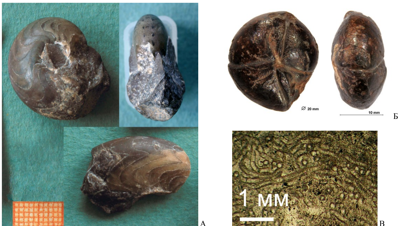
Рис. 3.34. Верхний девон. Аммониты (гониятиты): А – Manticoceras intumescens , раковины, доманиковый горизонт, Красноярский р-н, СОИКМ, фото Д.В. Варенова; Б – Cheiloceras amblylobum , ядро, фамен, Франция (по: Le coin ..., 2025). Цианопрокариоты, колонии: В – Girvanella sp., фран, Урал (по: Анфимов, 2015).
