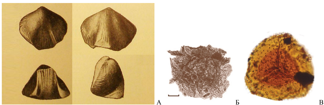
Рис. 3.21. Девон. А – брахиоподы: Ladogia triloba , раковина, пашийский горизонт, с. Берёзовка (Шигонский р-н) (по: Новожилова, 1955). Плауновидные, споры: Б – Densosporites [ D. meyeræ ], тиманский горизонт, Коми (по: Тельнова, Шумилов, 2019), Calypptosporites [ C. proteus ], средний девон, Воронежская обл. (по: Щемелинина, 2013).
