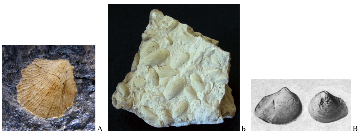
Рис. 5.37. Сосновская свита. Двустворчатые моллюски: А – Pseudomonotis permianus , отпечаток, Иса克林ский р-н; Б – Pseudobakewellia ceratophagaeformis , ядра, Винновские горы (Самарская лука); ИЭВБ, фото Д.В. Варенова; В – Schizodus rossicus , Архангельская обл., сакмарский ярус; ядра (по: Пермские морские ..., 1984).
