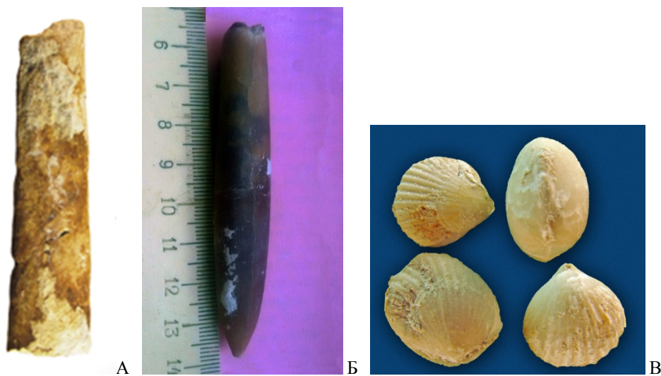
Рис. 8.32. Гулюшевская свита. А – аммонит Sciponoceras bohemicum ; фрагмент ядра, Саратовская обл. (по: Сельцер, 2018); Б – белемнит Goniosatama intermedius , ростр; В – брахиопода Orbirhynchia orbignyi , раковины. Шигонский р-н: СамГТУ (Б), ИЭВБ (В), фото В.П. Морова.
