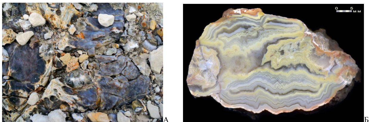
Рис. 5.46. Сосновская свита. А – корка халцедона на поверхности пласта гипса; Б – секрция агата. Сергиевский р-н. Фото И.В. Чихляева (А), ИЭВБ, фото Д.В. Варенова (Б).
