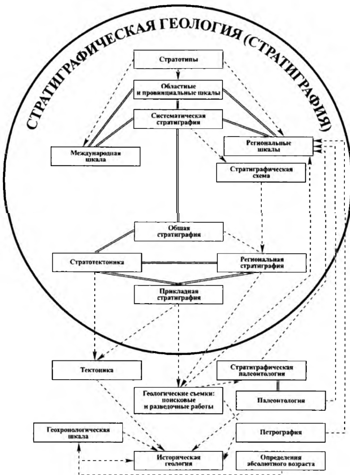
Рис. 1.2. Структура стратиграфической геологии (по: Егоян, 2012).
