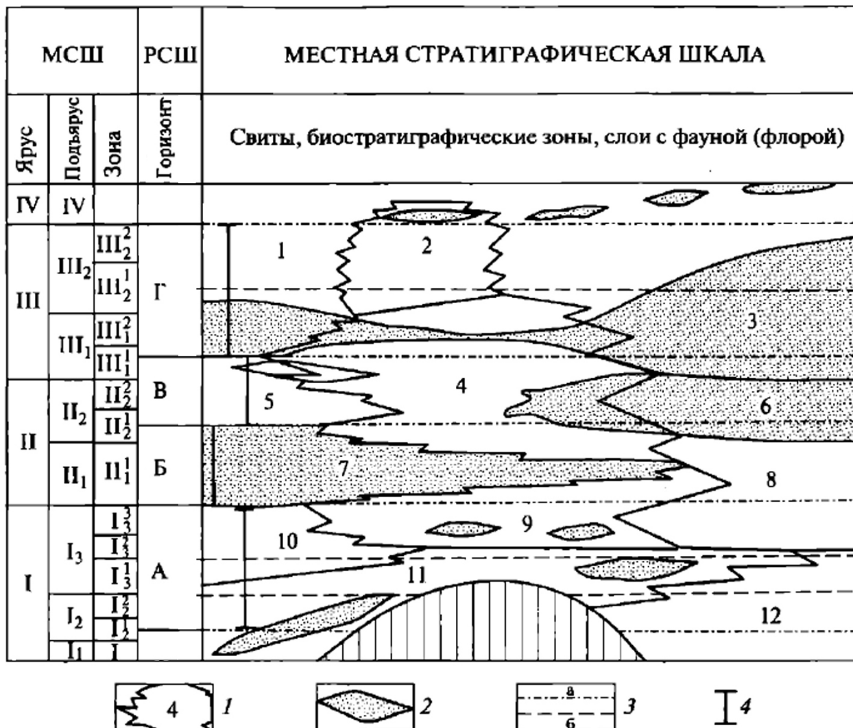
Рис. 1.11. Соотношение стратонов разных категорий и шкал: 1 – литостратоны; 2 – биостратоны; 3 – границы хроностратонов: а – горизонтов, б – хронозон; 4 – стратотипы горизонтов (по: Прозоровский, 2010).
