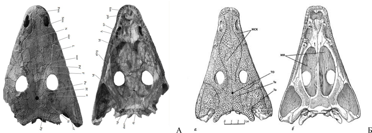
Рис. 6.12. Рыбинский горизонт. Черепа темноспондильных амфибий: А – Benthosuchus gusevae , Борский р-н (по: Новиков, 2018).; Б – B. sushkini , Ярославская обл. (по: Новиков, 2012)
