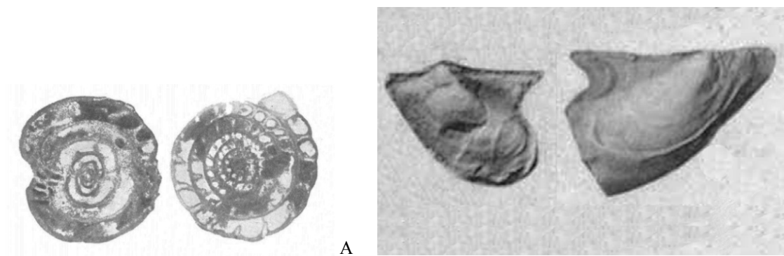
Рис. 5.16. Кунгурский ярус. А – фораминиферы Parastaffelloides pseudosphaeroidea , раковинки (сильно увел.), Пермская обл. (по: Дуткевич, 1934); Б – двустворчатый моллюск Pseudobakewellia antiquaeformis , Коми; створки раковин (по: Пермские морские ..., 1984).
