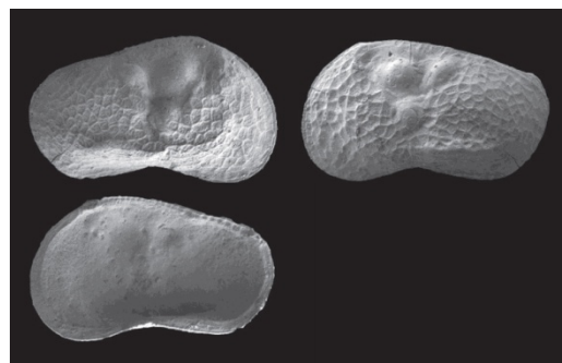
Рис. 11.3. Акчагыльский региоярус. Остракоды: Limnocythere alveolata , раковина (увел.), Азербайджан (по: Richards et al., 2018).
