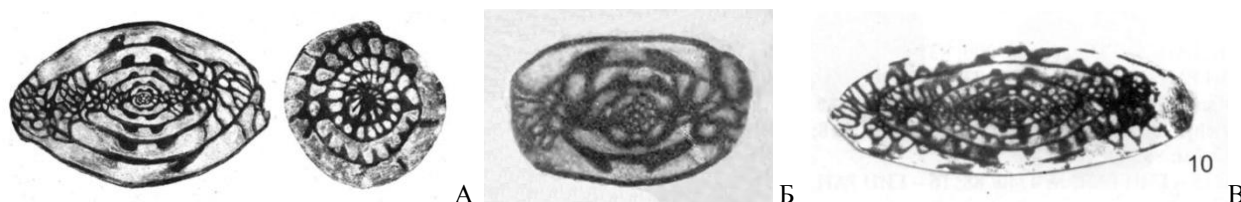
Рис. 4.49. Каширский горизонт. Фораминиферы, сечения (сильно увел.): А – Priscoidea priscoidea , гор. Сызрань, гор. Жигулёвск (по: Раузер-Черноусова, 1938), Б – Schubertella magna , Волгоградская обл. (по: Путря, 1956), В – Hemifusulina communis , Московская обл. (по: Средний карбон ..., 2001).
