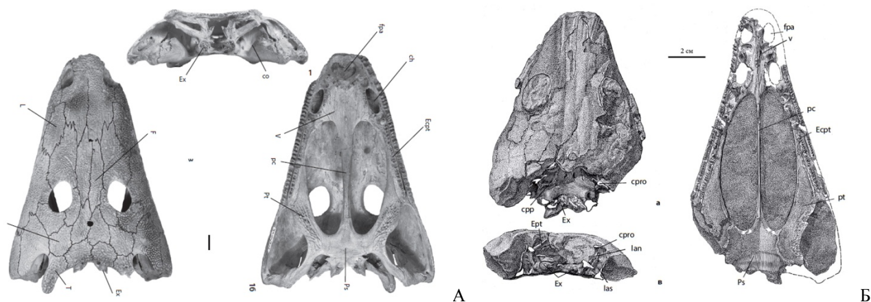
Рис. 6.17. Оленёкский ярус. Черепа темноспондильных амфибий: А – Wetlugasaurus angustifrons , слудкинский горизонт, Ярославская обл; Б – Angusaurus succedaneus , усть-мысльский горизонт, Алексеевский р-н. (по: Новиков, 2018).
