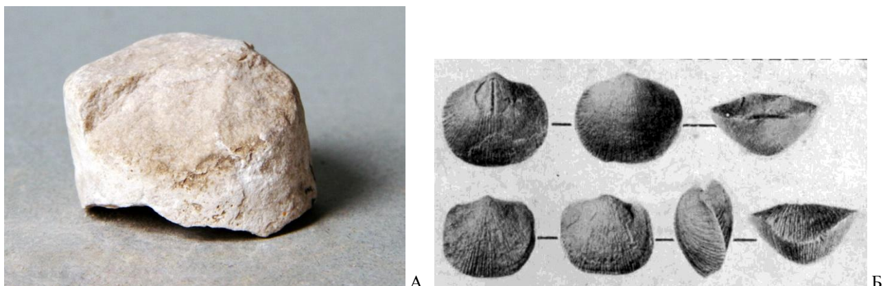
Рис. 4.4. Упинский горизонт. А – известняк (кern с глуб. 2752 м), Ореховская опорная скважина, СОИКМ; Б – брахиоподы: Schizophoria upensis , раковины, Подмоскowie (по: Сарычева, Сокольская, 1952).
