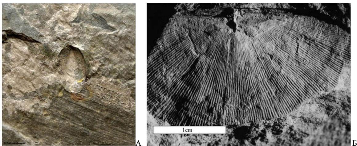
Рис. 4.14. Визе. Брахииподы: А – Lingula mytiloides , раковина, Чехия, фото: М. Pavla (по: Czech Paleontological ..., 2016); Б – Megachonetes zimmermanni , ядро створки, Польша (по: Kryza et al., 2011).
