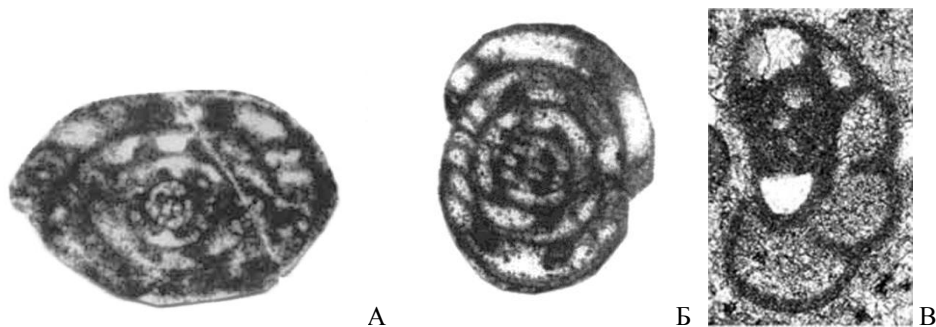
Рис. 4.39. Карбон. Фораминиферы, сечения (сильно увел.): А – Staffellaeformes staffellaeformis , Б – Pseudostaffella praegorskyi , средний карбон Турции (по: Dzhenchuraeva, Осууусу, 2007), В – Endothyra pseudobradyi , ассельский ярус Шпицбергена (по: Blazejowski, 2009).
