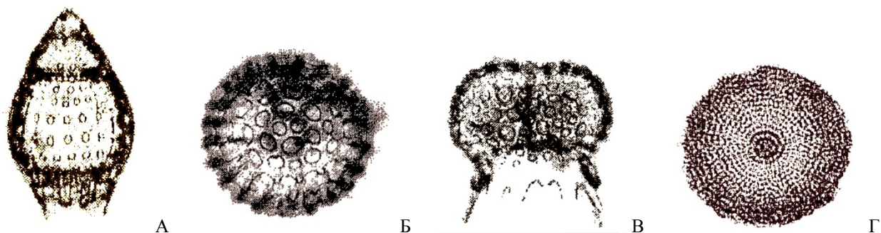
Рис. 9.9. Сызранская свита. Радиолярии: А – Buryella tetradica , Б – Entapium piriferum , В – Dorcadospyrus confluentis , Г – Spongotrochus pulcher , скелеты. Ульяновская обл. (А); Балашейское месторождение опок (Б-Г) (по: Козлова, 1999) (сильно увел.).
