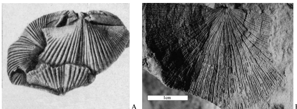
Рис. 4.28. Тарусский горизонт. Брахиоподы: А – “ Angiospirifer ” venevianus , ядра, Подмосковьё (по: Сарычева, Сокольская, 1952); Б – Schuchertella portlockiana , ядро створки, вие Польши (по: Haydukiewicz, Muszer, 2002).
