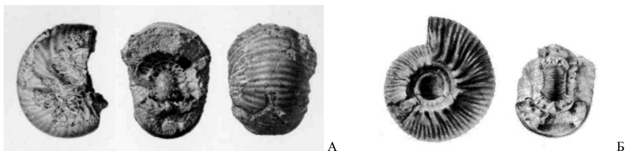
Рис. 8.7. Валанжинский ярус. Аммониты: А – Nikitinoceras ribkinianus , Рязанская обл. (по: Богословский, 1902), Б – Polyptychites gravesiformis , Кашпирский разрез (по: Pavlow, Lamplugh, 1892). Раковины и сечения.
