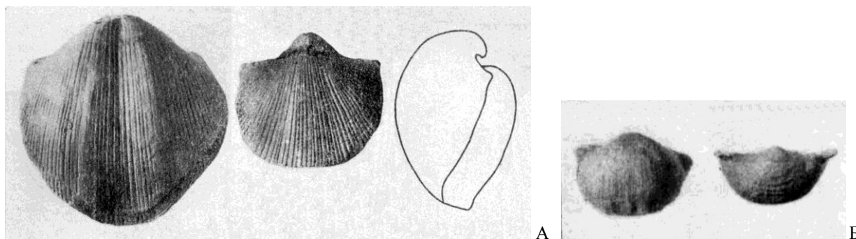
Рис. 4.48. Московский ярус. Брахиоподы: А – Choristites sowerbyi , Б – Kozlowskia kaschirica , раковины. Подмоскowie (по: Сарычева, Сокольская, 1952).
