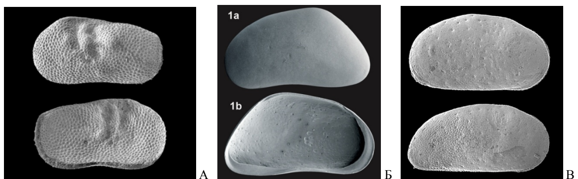
Рис. 11.8. Аккулаевская свита. Остракоды (створки, увел.): А – Ilyocypris bradyi , Б – Fabaeformiscandona balatonica , Б – Cyprideis torosa . Азербайджан (по: Richards et al., 2018) (А, Б), квартал Германии (по: Fuhrmann R., 2012) (Б).
