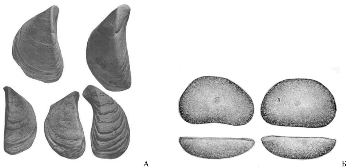
Рис. 10.4. Акчагыльский регионарус. Двустворчатые: А – Dreissena polymorpha , раковины, Башкортостан (по: Яхимович и др., 2000). Остракоды: Б – Cyprina candonaeformis , раковины (сильно увел.), верхний плиоцен – гелазий Омской обл. (по: Казьмина, 1975).
