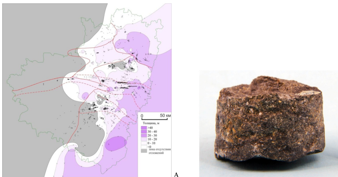
Рис. 3.9. Воробьёвский горизонт. А – распространение и мощность (по: Потёмкин, 2015). Б – гравелит (кern с глуб. 3780 м), Ореховская опорная скважина (Алексеевский р-н). СОИКМ.
