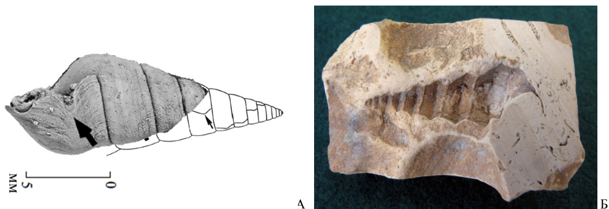
Рис. 5.38. Сосновская свита. Гастроподы: А – Arribazona lata , ПИН (по: Mazaev, 2017); Б – Goniasma sp., отпечаток, Винновские горы (Самарская лука). ИЭВБ, фото Д.В. Варенова.
