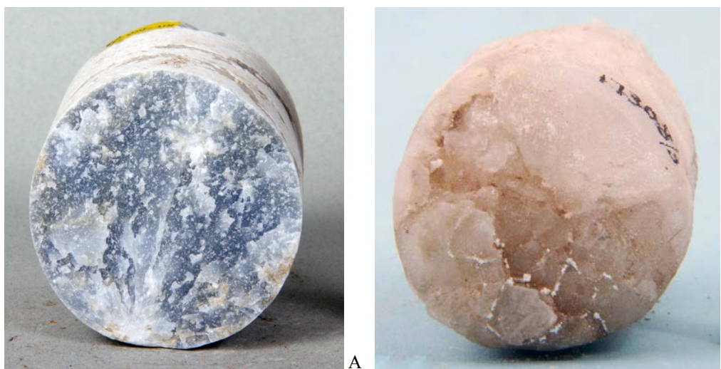
Рис. 5.17. Иренский горизонт. А – ангидрит (кern с глуб. 240 м), р-н с. Сухарь-Матак (Исаклинский р-н); Б – каменная соль, kern (глуб. 643 м), р-н с. Ореховка (Алексеевский р-н). СОИКМ, фото Д.В. Варенова.
