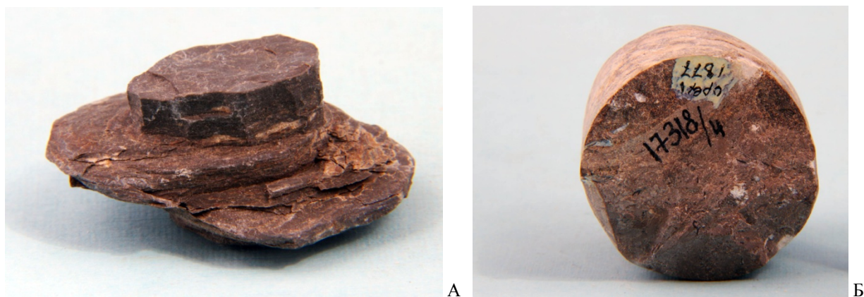
Рис. 3.15. Ардаковский горизонт. А – глина (кern с глуб. 3727 м); Б – известняк (кern с глуб. 3723 м). Ореховская опорная скважина; СОИКМ.
