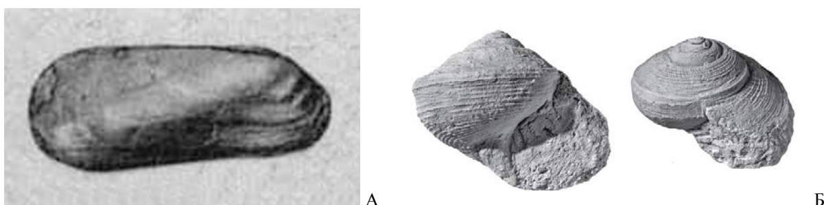
Рис. 5.31. Немдинский горизонт. А – двустворчатый моллюск Verneuilnodon pallasii , ядро, Коми, уфимский ярус (по: Пермские морские ..., 1984); Б – гастропода Glabrocingulum lebedewi , Камышлинский р-н (по: Mazaev, 2018).
