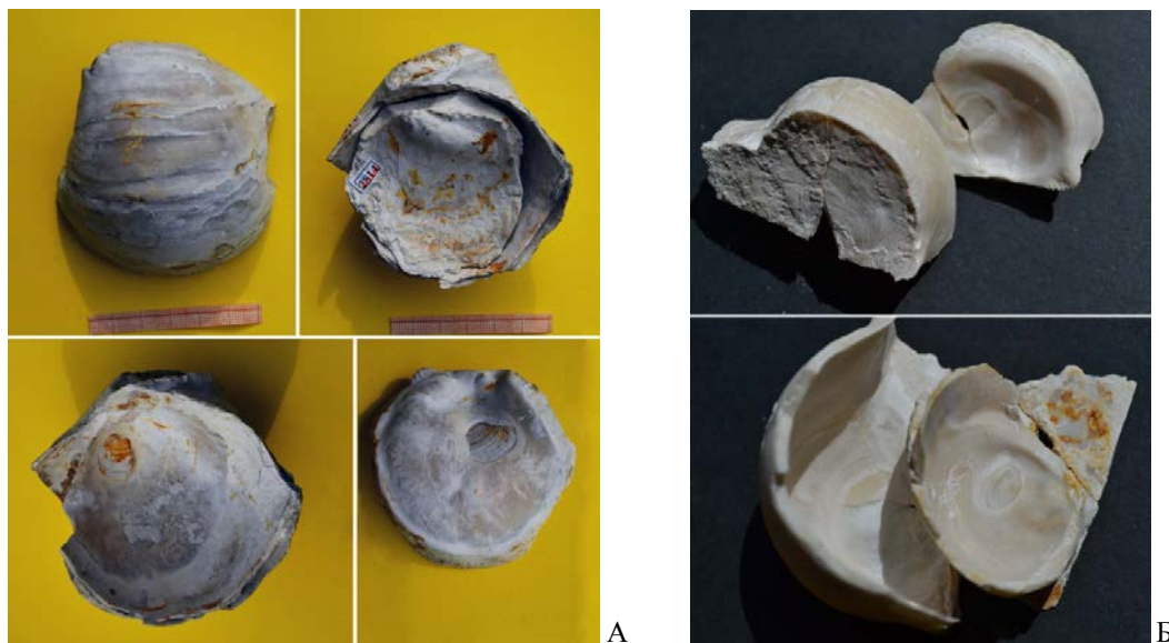
Рис. 8.47. Кампанский ярус. Двустворчатый моллюск Pycnodonte vesicularis : раковины со слабо (А) и сильно (Б) деформированной за счёт прикрепления макушкой. Левая створка выпуклая, правая – вогнутая. Разрез Подвалье. ИЭВБ, фото В.П. Морова.
