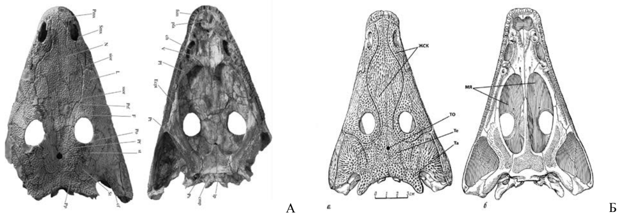
Рис. 10. Рыбинский горизонт. Черепа темносpondильных амфибий: А – Benthosuchus gusevae , Борский р-н; Б – Benthosuchus sushkini , Ярославская обл. [4, 5].
