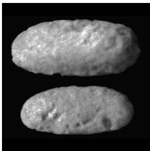
Рис. 4. Вохминский горизонт. А – конгломерат на основе гальки уральских пород с кальцитовым цементом, близ с. Подгорное (Борский р-н), СОИКМ, Фото Д.В. Варенова; Б – позвонки амфибии Tupilakosaurus sp., Оренбургская обл., фото Р.А. Гунчина.
