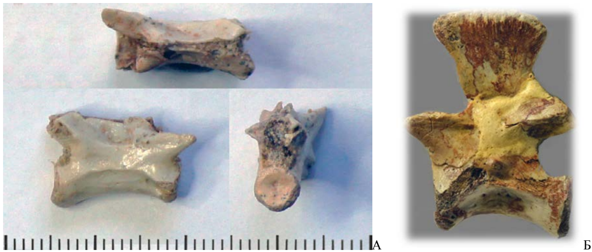
Рис. 11. Рыбинский горизонт. Позвонки рептилий: А – Microcnemus sp. (шейный), Б – Tsylosuchus samariensis ; Борский р-н. Фото Р.А. Гучина (А), ПИН РАН (Б).
