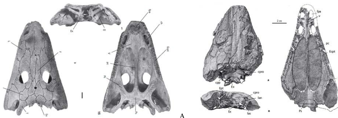
Рис. 14. Оленёкский ярус. Черепа темноспондильных амфибий: А – Wetlugasaurus angustifrons , слудкинский горизонт, Ярославская обл; Б – Angusaurus succedaneus , усть-мыльский горизонт, Алексеевский р-н. [8]
