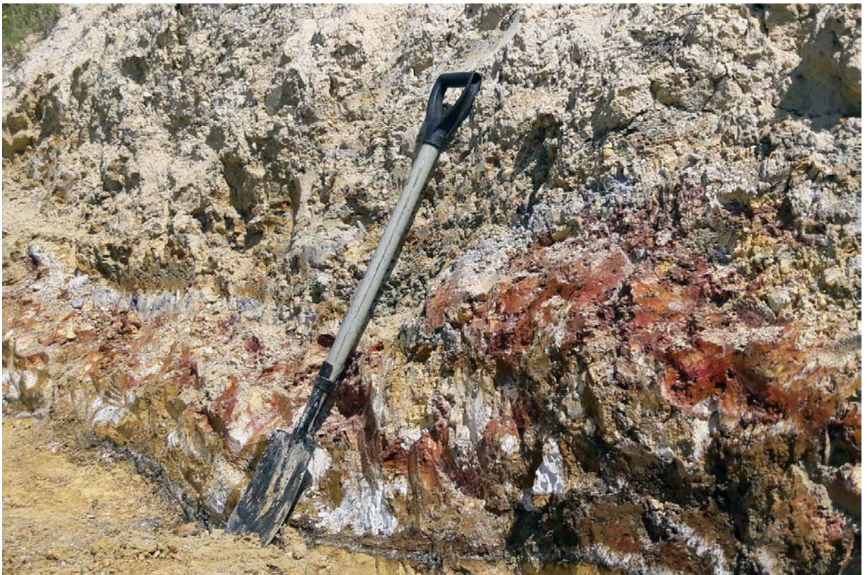
Рис. 1. Триас-нижнеюрская кора выветривания карбонатных пород казанского яруса пермской системы с минерализацией алунином. Самарская лука, с. Ермаково. Фото с геологической практики студентов СамГТУ, 2019.
