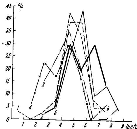
Рис. 22. Кривые изменчивости отношения ширины синуса (Шс) к ширине раковины (Ш) L. stuckenbergi из разных местонахождений
