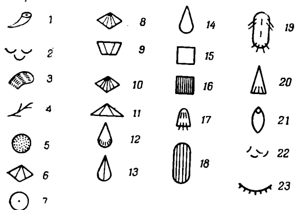
Рис. 25. Схема относительного обилия фауны II элемента байтуганских слоев (с. Камышла — комплекс I)
