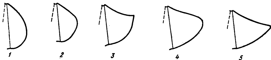
Рис. 8. Очертания боковых частей раковины рода Licharewia 1—3 — L. rugulata , 4—5 — L. stuckenbergi
