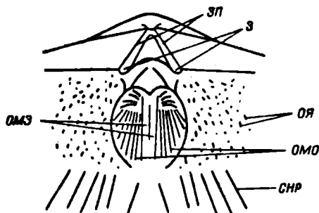
Рис. 6. Схема внутреннего строения брюшной створки рода Licharewia
