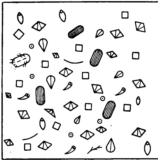
Рис. 33. Схема относительного обилия фауны III элемента байтуганских слоев (с. Камышла, комплекс III). Условные обозначения на рис. 25
