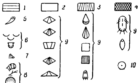
Рис. 26. Схема систематического (1) и экологического состава (2) фауны байтуганских слоев (с. Камышла — комплекс I)
