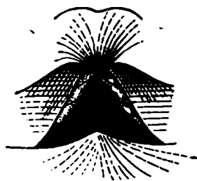
Рис. 16. Псевдодельтидий представителей рода Licharewia
