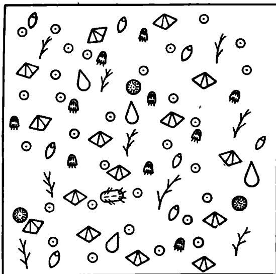
Рис. 30. Схема относительного обилия фауны II элемента байтуганских слоев (с. Шугурово, комплекс II). Условные обозначения на рис. 25
