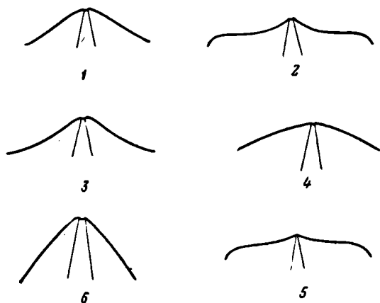
Рис. 14. Очертания заднего края:
