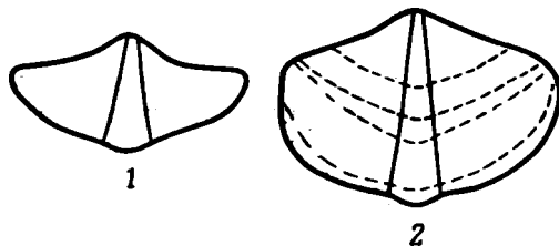
Рис. 10. Licharewia stuckenbergi 1 — молодой экземпляр, 2 — взрослый экземпляр
