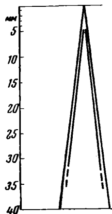
Рис. 18. Схема ребристости синуса представителей рода Licharewia
