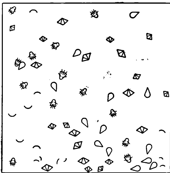
Рис. 27. Расположение фауны в вертикальной стенке обнажения (50×50 см). С. Камышла, обн. 1, сл. 4а. Условные обозначения на рис. 25
