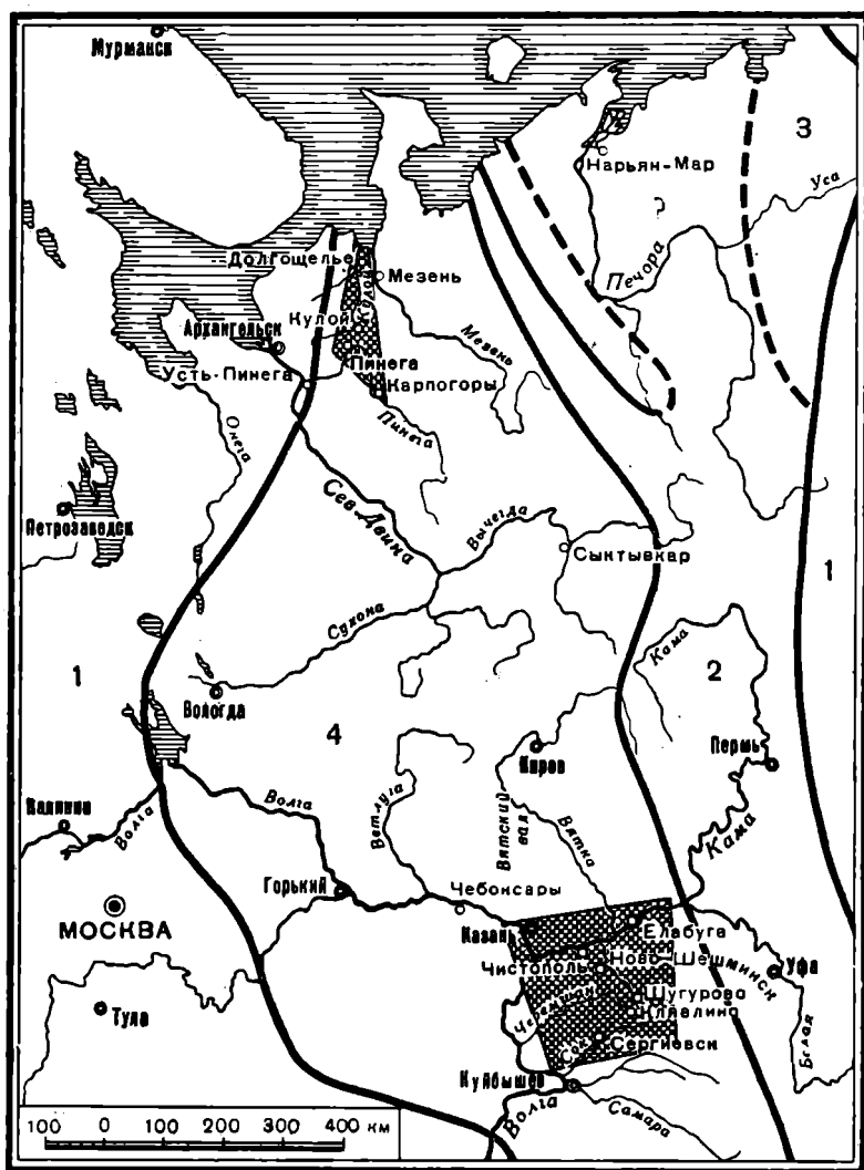
Рис. 1. Палеогеографическая карта раннеказанского моря Русской платформы (по А. Д. Архангельскому, 1932)
