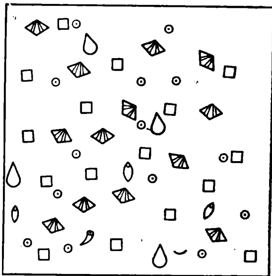
Рис. 36. Схема относительного обилия фауны III элемента камышлинских слоев (Берсут, комплекс IV). Условные обозначения на рис. 25
