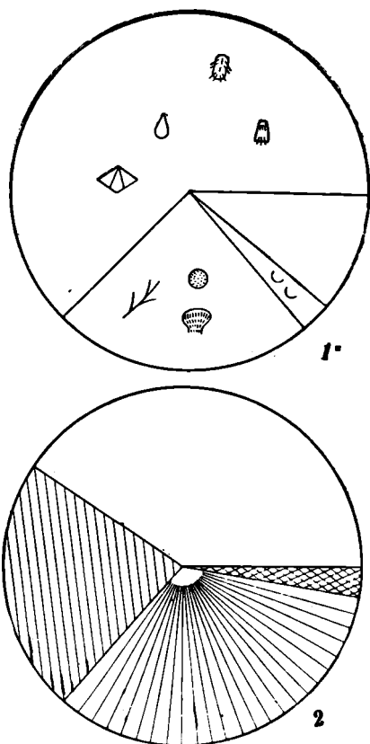
Рис. 31. Схема систематического (1) и экологического (2) состава фауны II элемента байтуганских слоев (с. Шугурово, комплекс II). Условные обозначения на рис. 26
