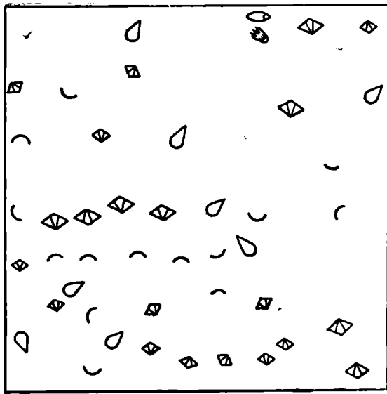
Рис. 29. Расположение фауны в вертикальной стенке обнажения (50×50 см). С. Камышла, обн. 1, сл. 1. Условные обозначения на рис. 25
