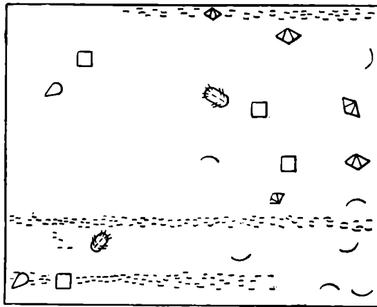
Рис. 34. Расположение фауны в вертикальной стенке обнажения (50×50 см). С. Камышла, обн. 5, сл. 3. Условные обозначения на рис. 25
