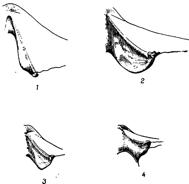
Рис. 20. Различная форма боковой поверхности зубных пластин представителей рода Licharewia
