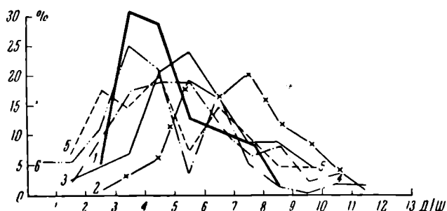
Рис. 23. Кривые изменчивости отношения длины раковины к ее ширине у L. rugulata
