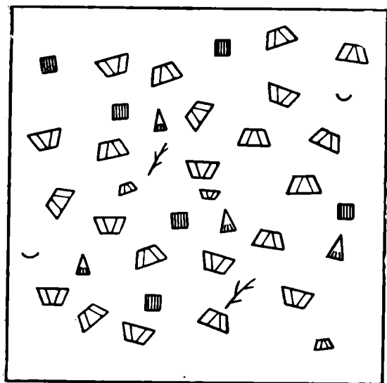
Рис. 38 Схема относительного обилия фауны слоев с P. keyserlingi по р. Кулою. Условные обозначения на рис. 25
