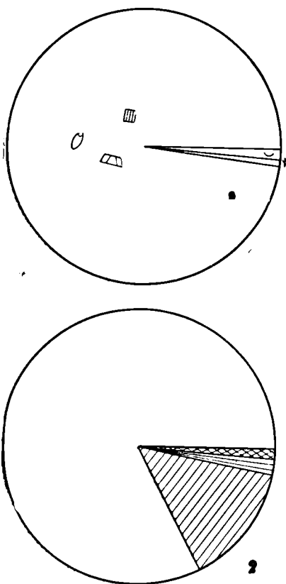
Рис. 39. Схема систематического (1) и экологического состава (2) фауны нижней части казанского яруса по р. Кулою, обл. 7. Условные обозначения на рис. 26
