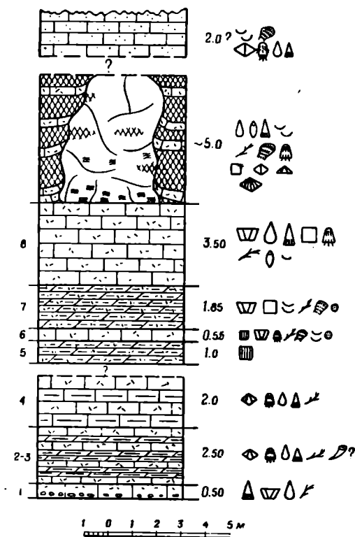
Рис. 4. Разрез нижнеказанских отложений у с. Долгощелье на р. Кулой. Условные обозначения см. на рис. 2
