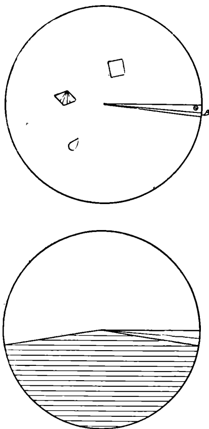
Рис. 37. Схема систематического (1) и экологического (2) состава фауны III элемента камышлинского цикла (Пр. Берсут, комплекс IV). Условные обозначения на рис. 26
