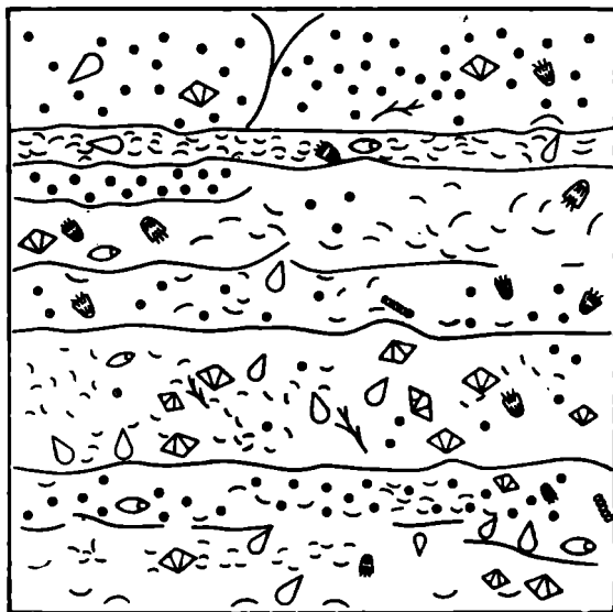
Рис. 32. Расположение фауны в вертикальной стенке обнажения (50×50 см). С. Шугурово, обн. 7, сл. 5. Условные обозначения на рис. 25
