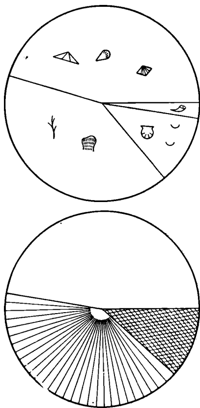
Рис. 41. Схема систематического и экологического состава фауны казанских отложений в глинах по склонам биогермов на р. Пинеге, обн. 12. Условные обозначения на рис. 26
