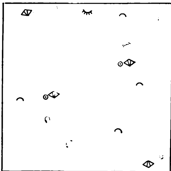
Рис. 28. Расположение фауны в вертикальной стенке обнажения (50×50 см). С. Камышла, обн. 1, сл. 3. Условные обозначения на рис. 25
