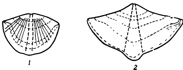
Рис. 12. Появление ушек на более ранних стадиях развития 1 — Permospirifer kulikovii , 2 — Licharewia grewinkii
