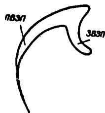
Рис. 19. Схема строения зубной пластины представителей рода Licharewia
