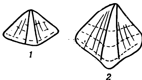
Рис. 9. Licharewia latiareata 1 — молодой экземпляр — с. Шугурово, 2 — взрослый экземпляр — Архангельская область
