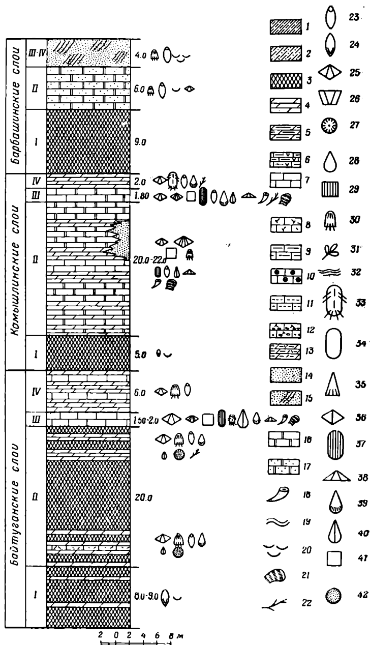
Рис. 2. Сводный разрез нижнеказанских отложений по р. Сок
