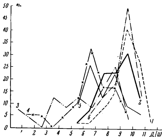
Рис. 21. Кривые изменчивости отношения длины раковины (Д) к ширине (Ш) у L. stuckenbergi из разных местонахождений
