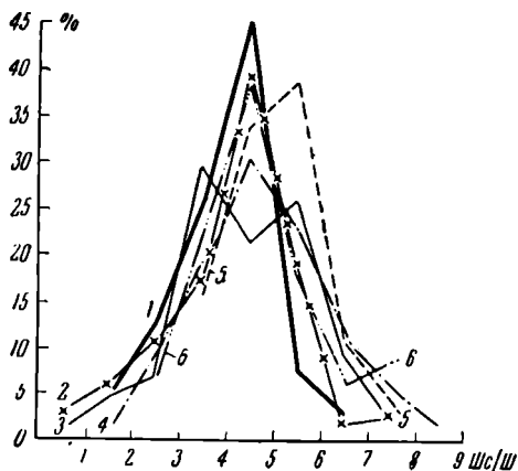
Рис. 24. Кривые изменчивости отношения ширины синуса к ширине раковины у L. rugulata из разных местонахождений. Условные обозначения см. на рис. 23
