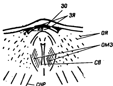
Рис. 7. Схема внутреннего строения спинной створки рода Licharewia
