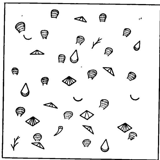
Рис. 40. Схема относительного обилия фауны в глинах, покрывающих склоны биогермов на р. Пинеге. Условные обозначения на рис. 25
