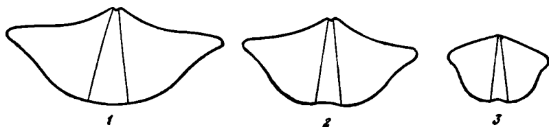
Рис. 11. Форма ушек у различных представителей подсем. Licharewinae 1 — Licharewia grewinkii , 2 — L. stuckenbergi , 3 — Permospirifer kulikovii
