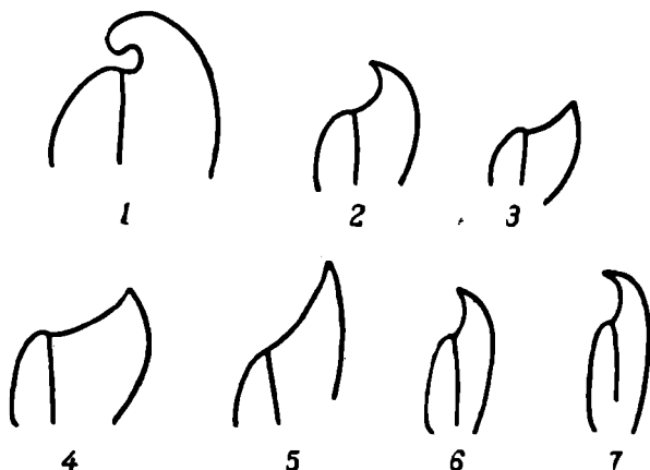
Рис. 13. Форма макушки (вид сбоку)
