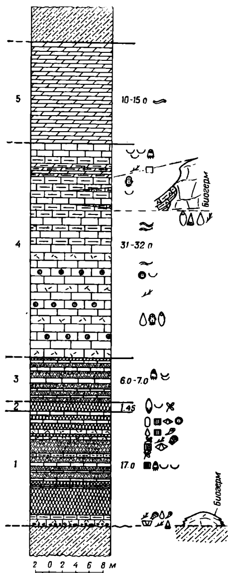
Рис. 3. Сводный разрез нижнеказанских отложений по р. Пинеге. Условные обозначения см. на рис. 2
